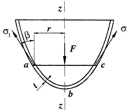
Рисунок 16. Схема оболочки вращения
