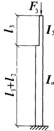
Рисунок И.1. Схема двухступенчатой колонны (а) и условные схемы нагружений при приложении сил F_1 , F_2 и F_3 соответственно к нижнему (б), среднему (в), верхнему (г) участкам
