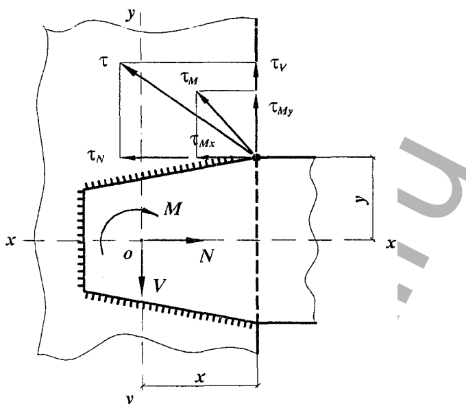
Рисунок 21. Расчетная схема сварного соединения
