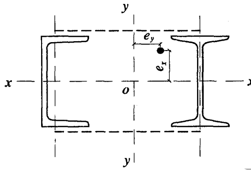
Рисунок 12. Схема сквозного сечения стержня из двух сплошнотенчатых ветвей
