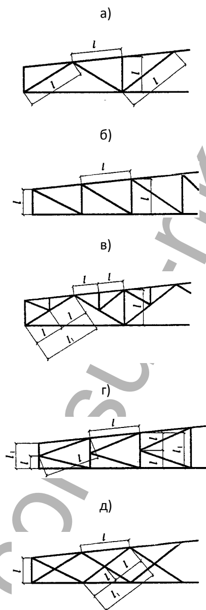
а - треугольная со стойками; б - раскосная; в - треугольная со шпренгелями; г - полураскосная треугольная; д - перекрестная
