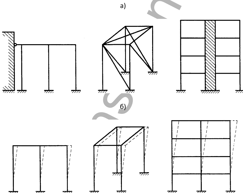
Рисунок 1. Схемы систем раскрепленных (а) и не раскрепленных от перемещений (б)
