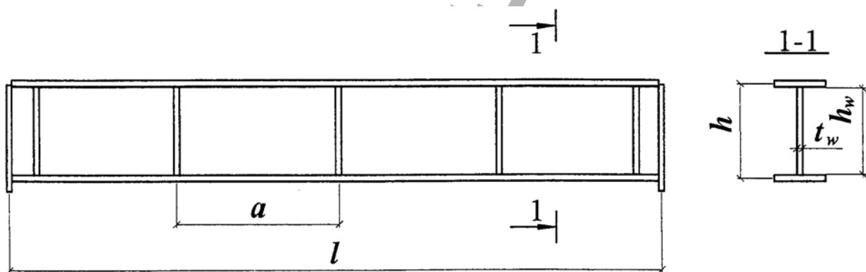
Рисунок М.1. Схема балки с гибкой стенкой
