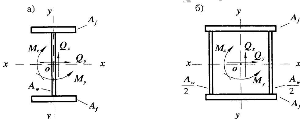
Рисунок 7. Схемы двутаврового (а) и коробчатого (б) сечений балок с действующими на них усилиями
