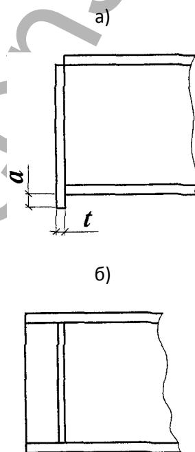
а - в торце с применением строжки; б - удаленного от торца с плотной пригонкой или приваркой к нижнему поясу
