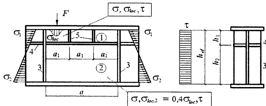
Рисунок 10. Схема балки, укрепленной поперечными (3), продольными (4) и промежуточными (5) ребрами жесткости
