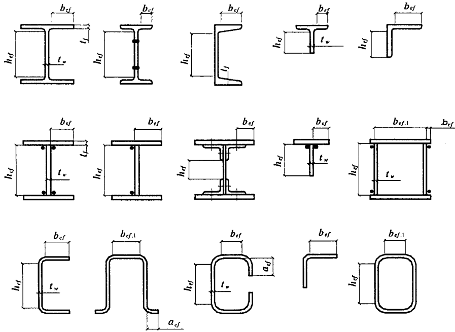
Рисунок 5. Расчетные размеры стенок, свесов полок, поясных листов в прокатных, составных и гнутых профилях
