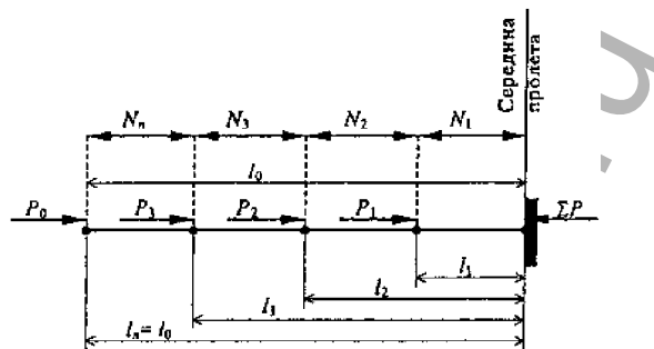
Рисунок Л.1. Расчетная схема сжатых участков пояса фермы
