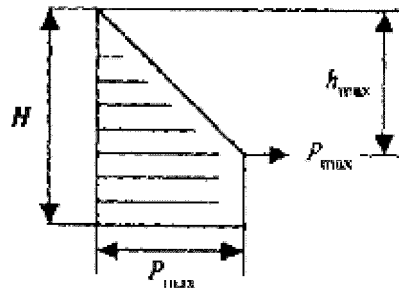
Рисунок 16.1. Расчетные эпюры бокового давления бетонной смеси
