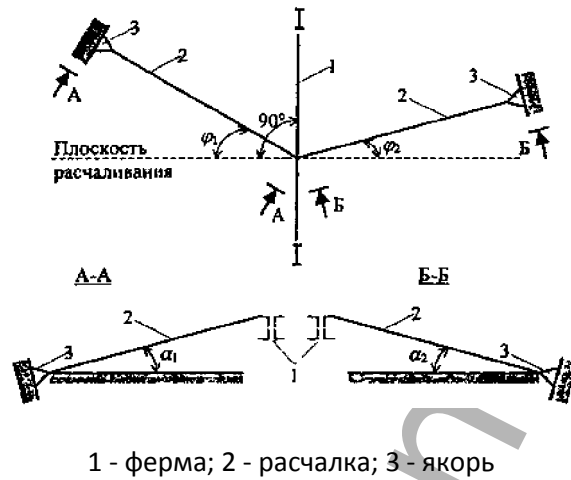
Рисунок Л.2. Схема раскрепления ферм расчалками
