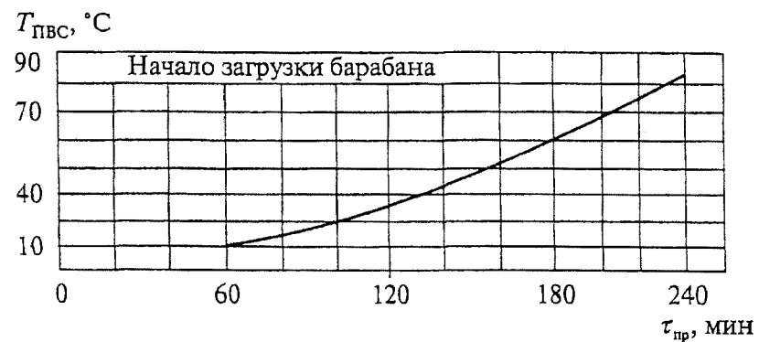
ГРАФИК НАГРЕВА ПАРОВОЙ ТРУБЧАТОЙ СУШИЛКИ
